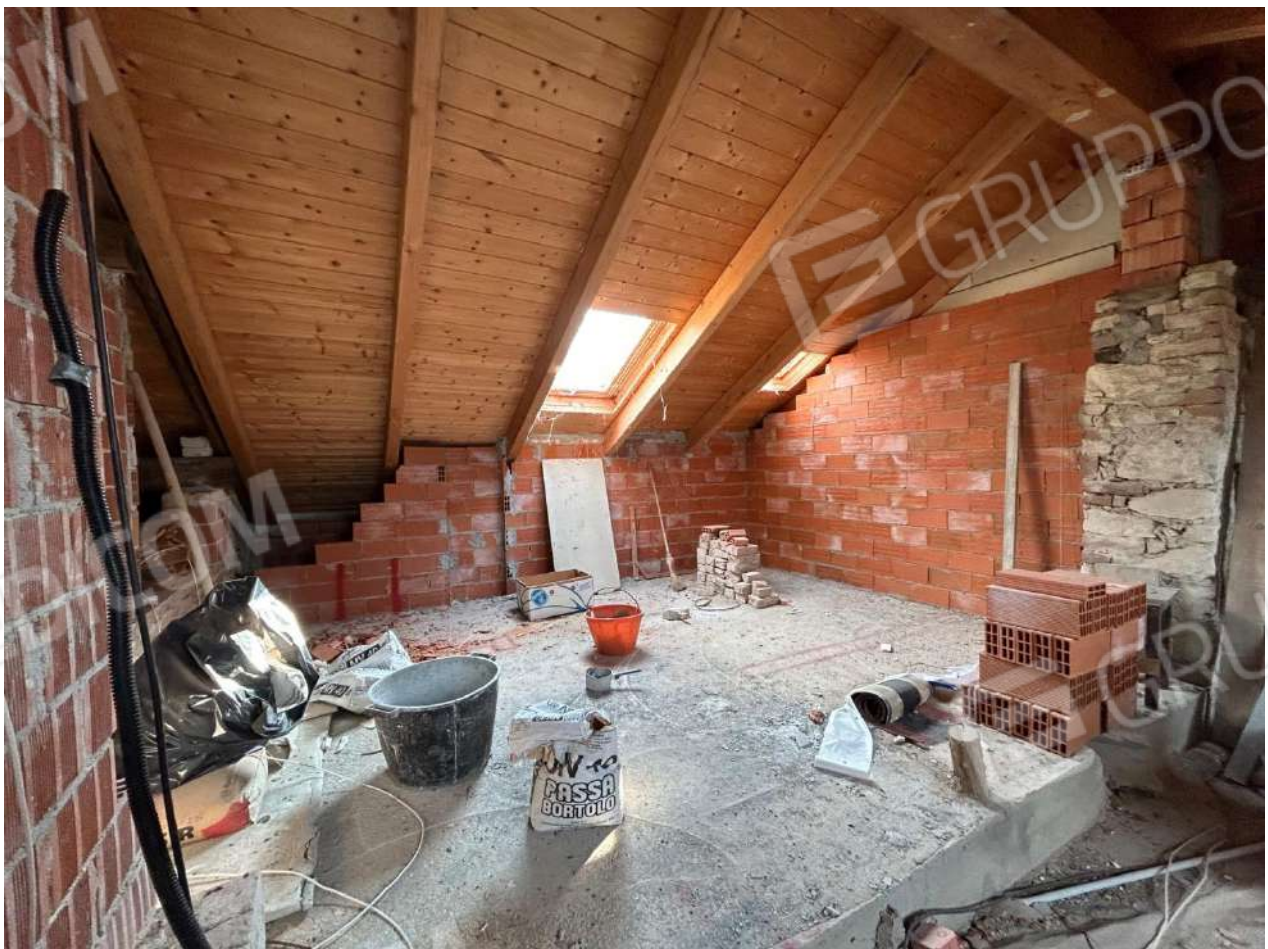
Sottotetto
