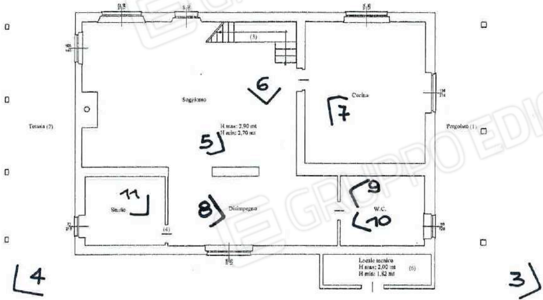
Pianta piano terreno - stato di rilievo
