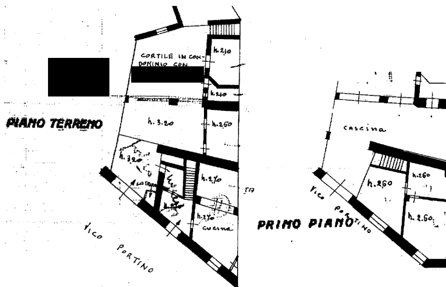
Planimetria catastale agli atti – stato legittimo
