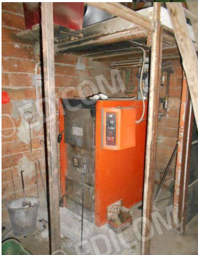
il generatore dell'impianto di riscaldamento alimentato a legna
