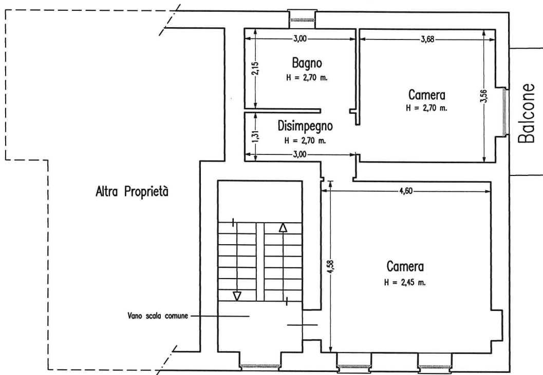
Piano Primo Scala 1:100
