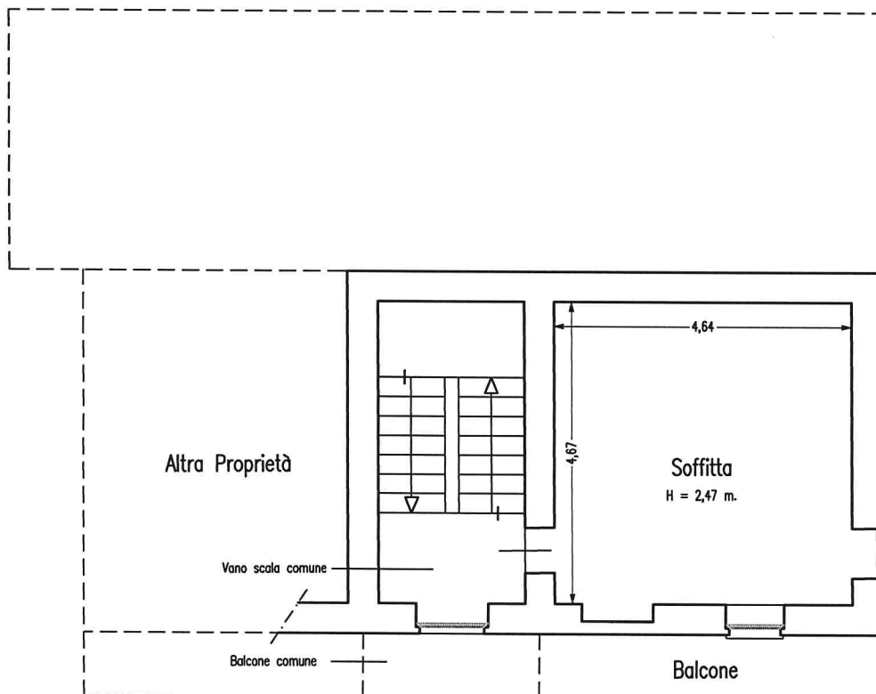
Piano Secondo Scala 1:100
