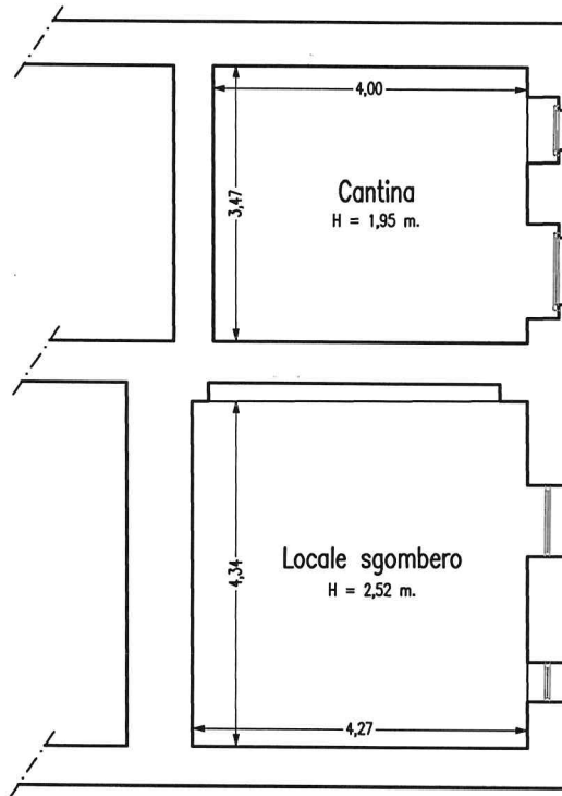
Piano Interrato Scala 1:100
