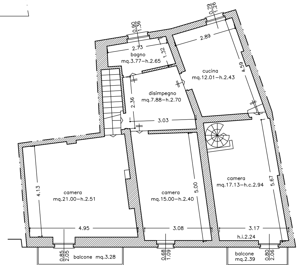
pianta piano primo situazione attuale
