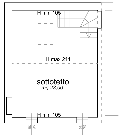
PIANO SOTTOTETTO (2°)
