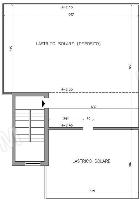
PIANO LASTRICO SOLARE
