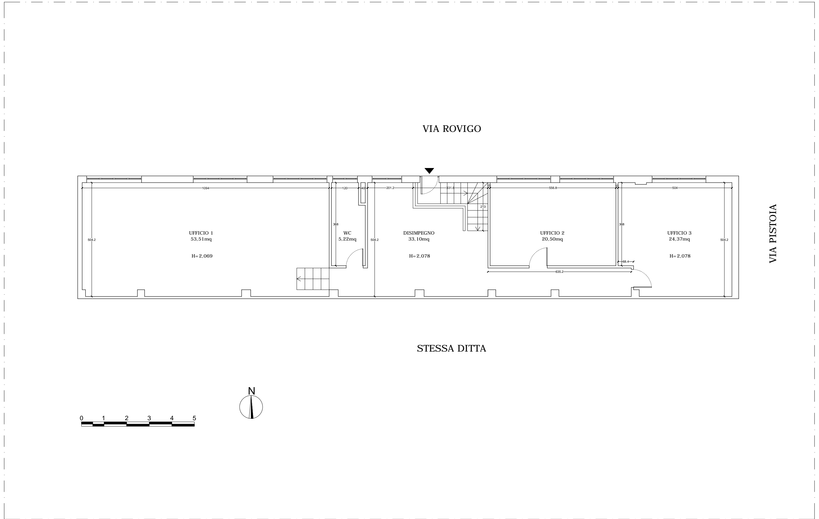
PIANTA PIANO 1° - STATO DI FATTO
