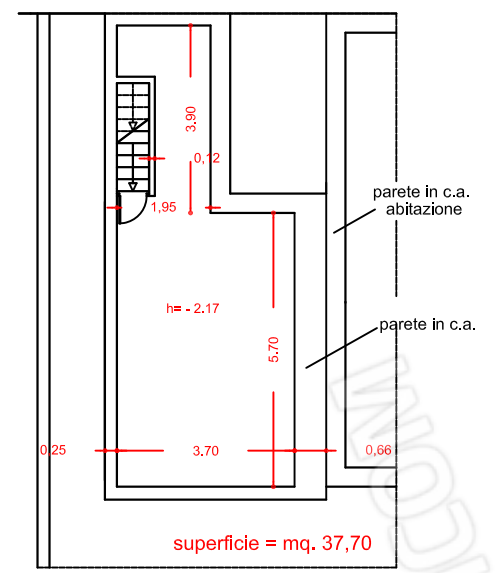
Piano interrato "Deposito"
