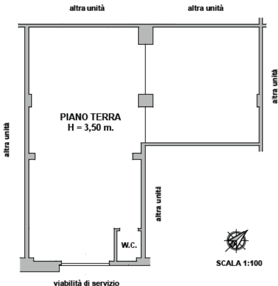
Fig. 2 - LOTTO 6 - Planimetria laboratorio artigianale foglio 76 - part. 620 - sub. 69
