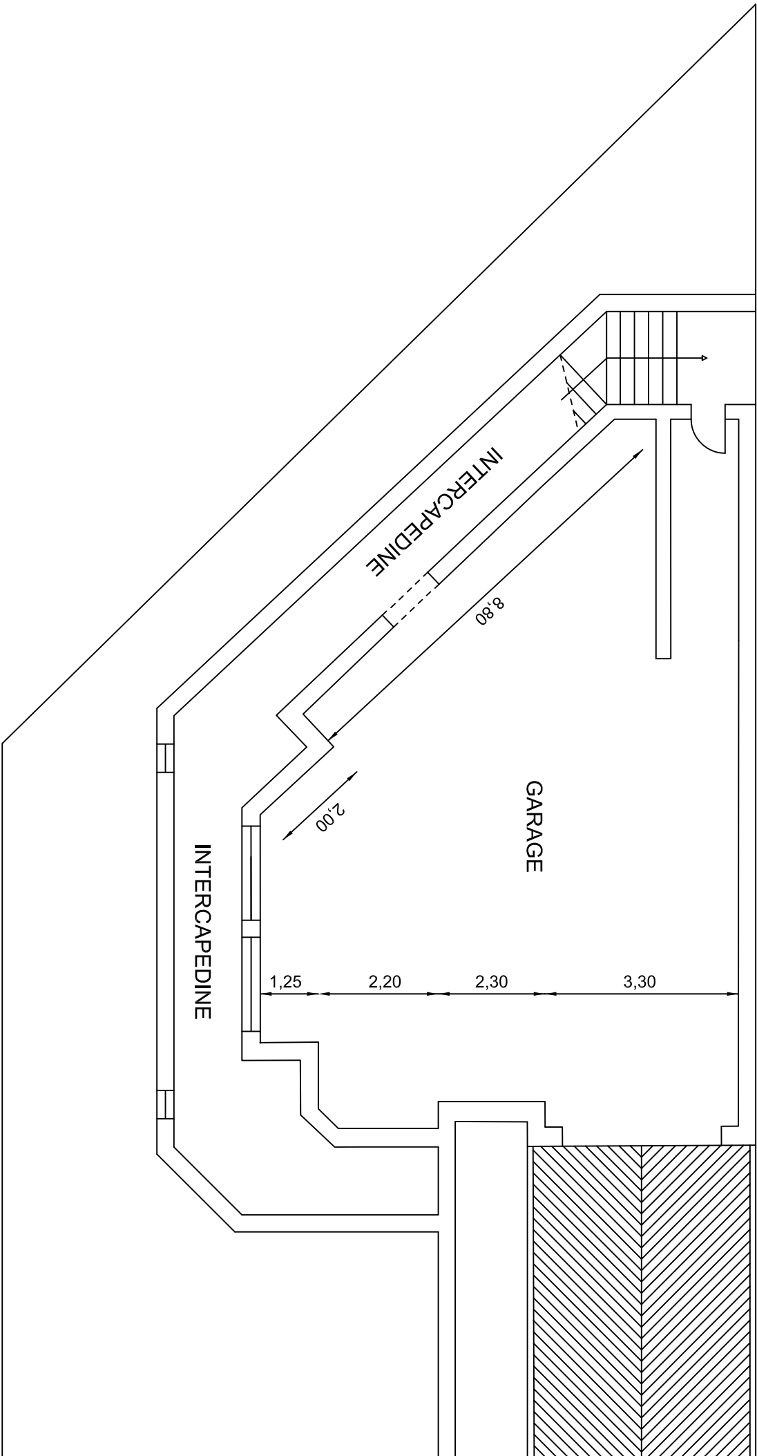
PIANTA PIANO SEMINTERRATO
