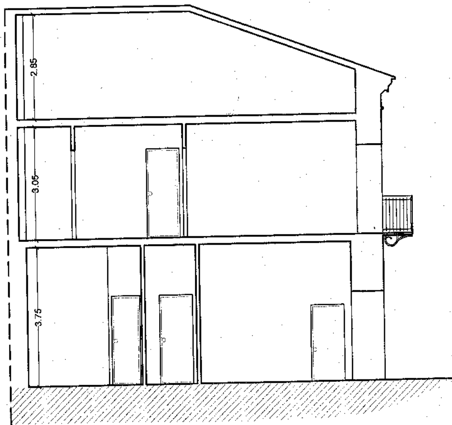
SEZIONE A-A
