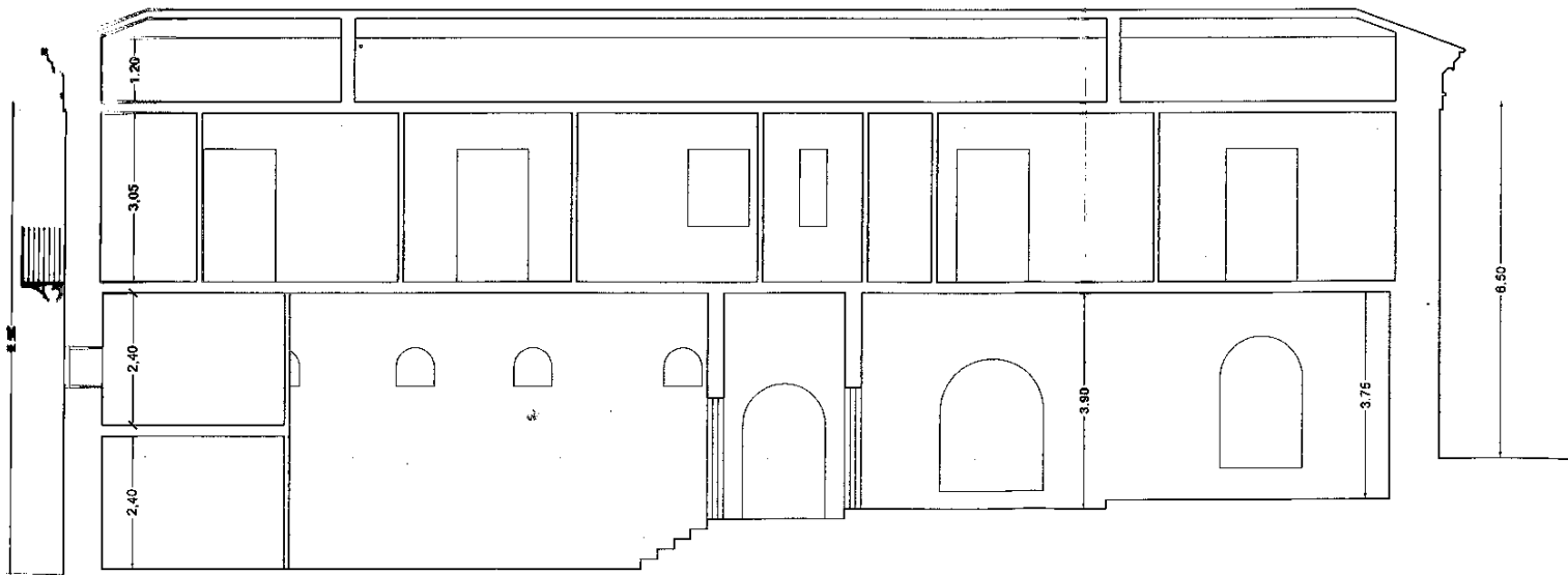
SEZIONE A-A
