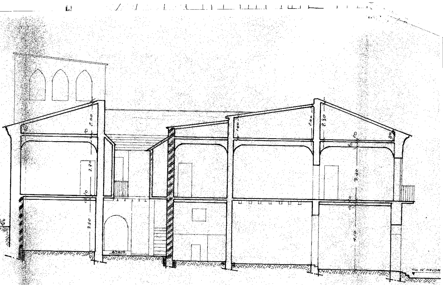
SEZIONE LONGITUDINALE
