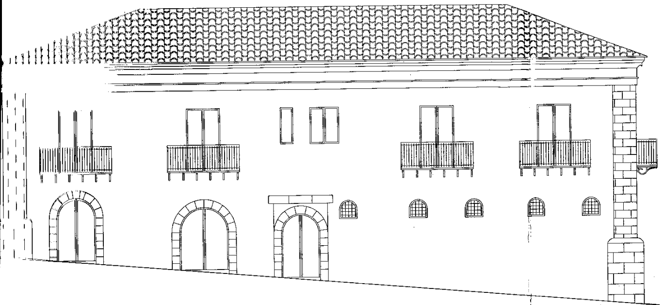
PROSPETTO SU VIA DI VINCENZO
