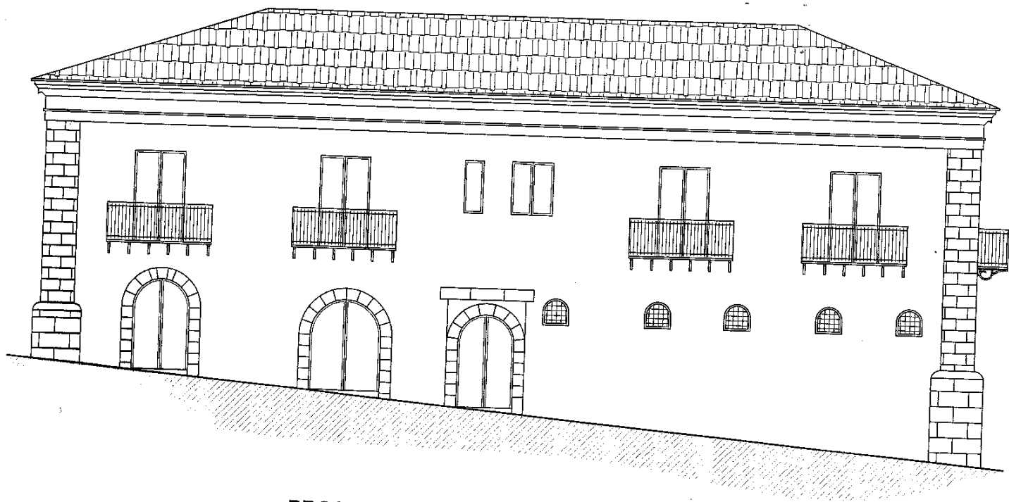
PROSPETTO SU VIA DI VINCENZO
