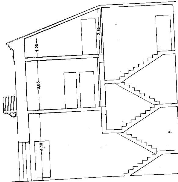
SEZIONE B-B
