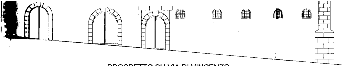
PROSPETTO SU VIA DI VINCENZO
