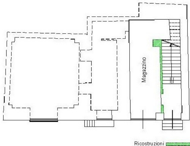
Sovrapposizione planimetria originaria e stato attuale piano terra quota m 0,00
