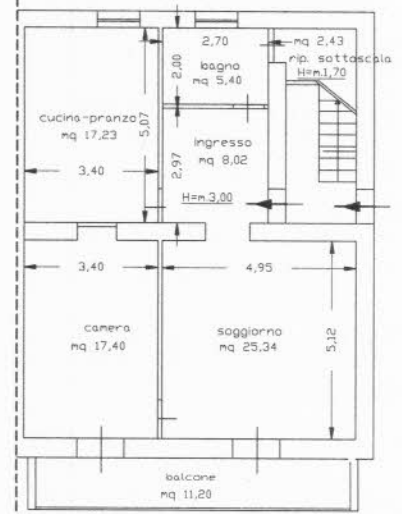
PLANIMETRIA STATO FUTURO VIA PERUGINO N.1, PORTO EMPEDOCLE F. 23 PART.297 SUB. 1 - 2
