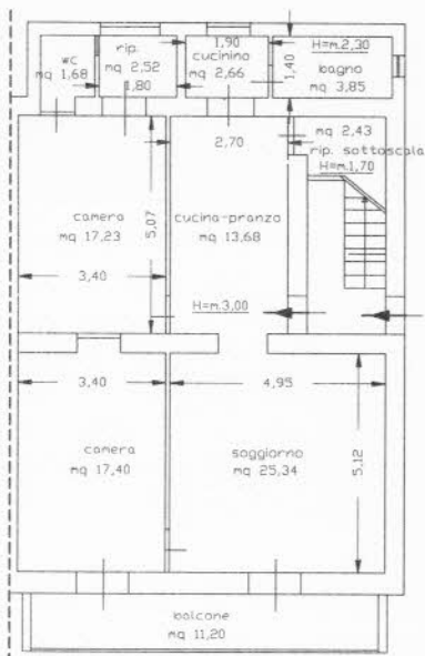
PLANIMETRIA STATO ATTUALE APPARTAMENTO AL PIANO TERRA VIA PERUGINO N.1, PORTO EMPEDOCLE F. 23 PART.297 SUB. 1 - 2
