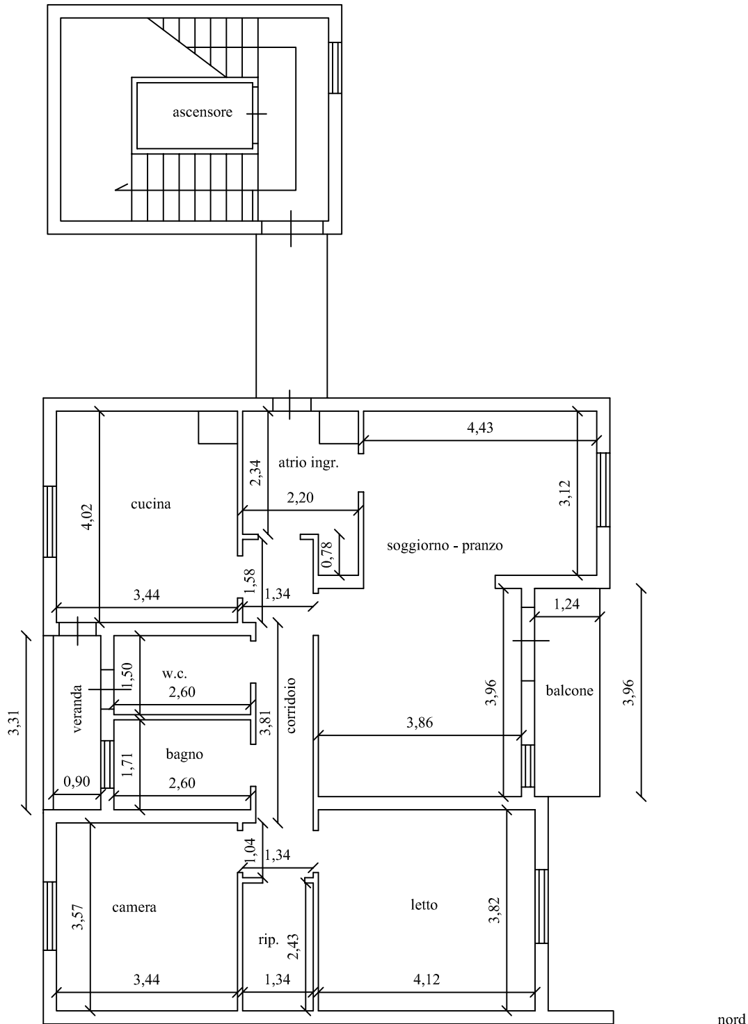
Pianta in scala 1:100 immobile in Porto Empedocle via Aldo Moro n. 8 torre otto in catasto al fg. 22 part. 673 sub. 27 piano undicesimo
