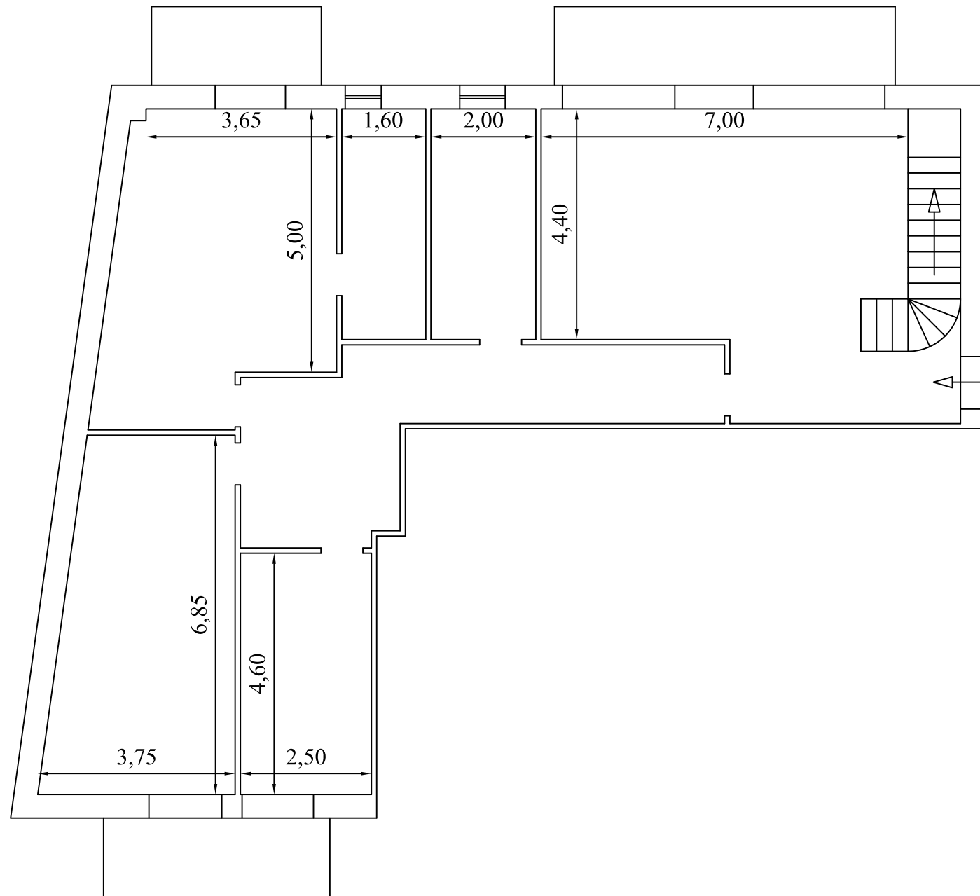
Secondo Piano H = 3,00 m.
