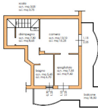
PIANO PRIMO
