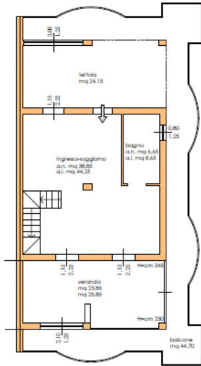
PIANO SECONDO
