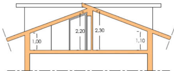
SEZIONE A-A'
