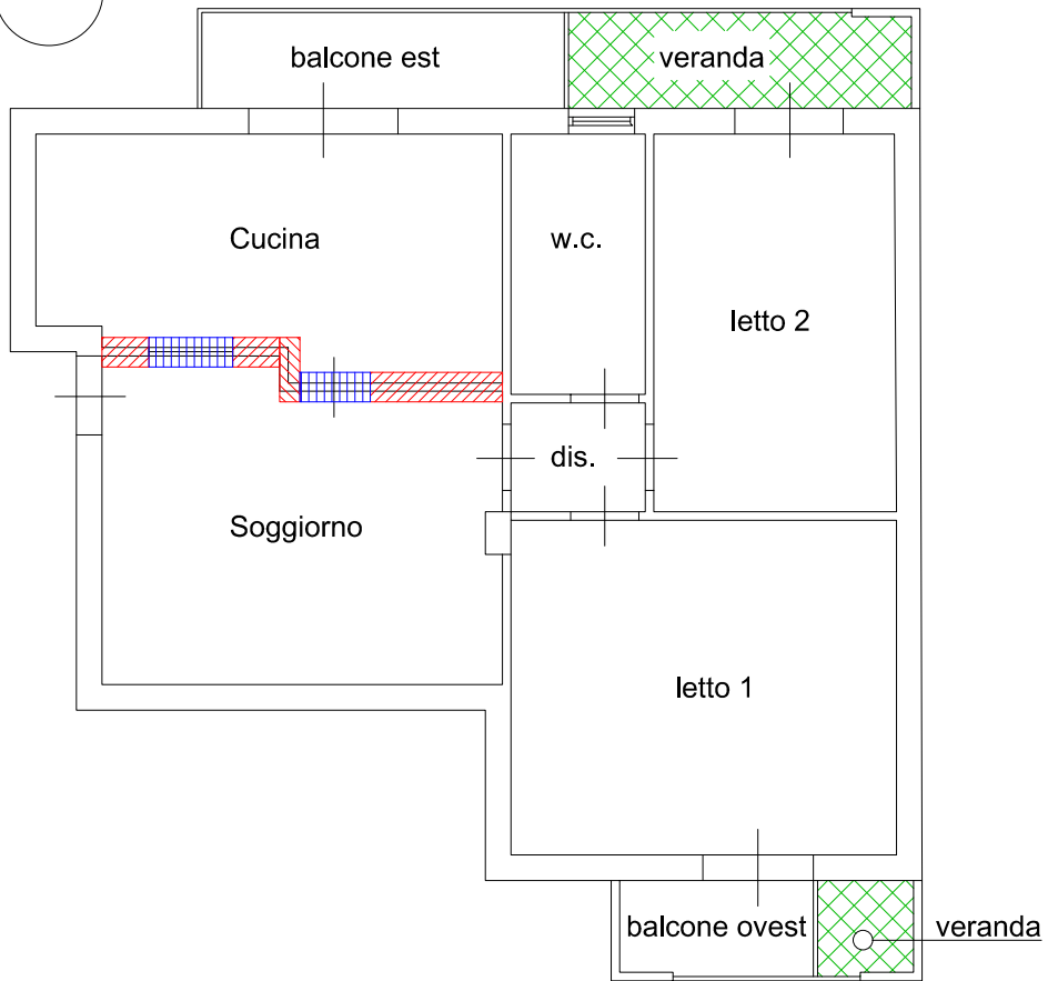
PIANTA PIANO SECONDO IMMOBILE - DIFFORMITA' TRA STATO DI FATTO E CATASTALE
