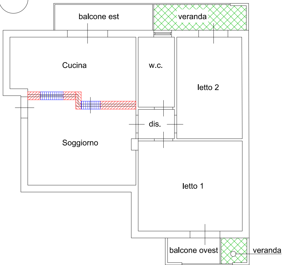
PIANTA PIANO SECONDO IMMOBILE - DIFFORMITA' TRA STATO DI FATTO E PROGETTO
