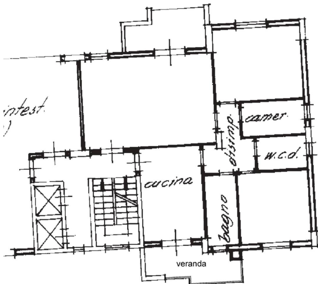
ALLEGATO N. 3 - Planimetria dello stato reale dei luoghi
