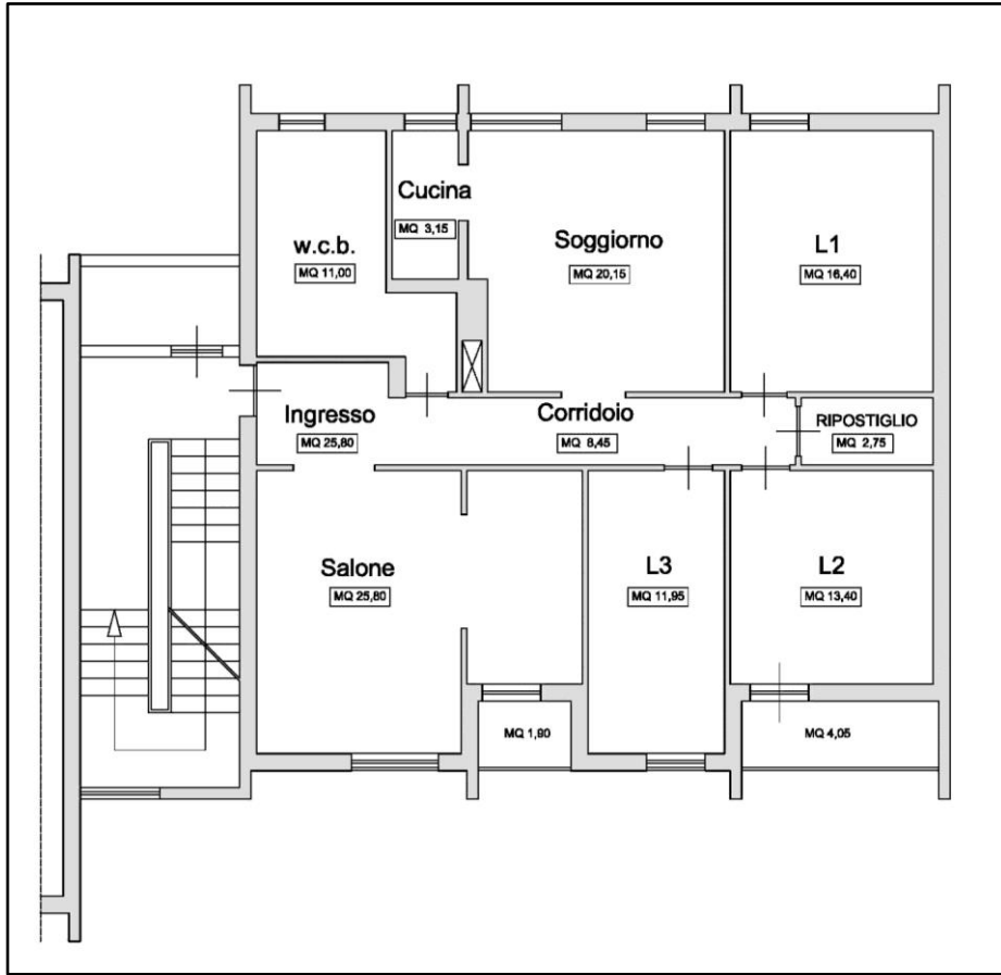
Planimetria dello stato attuale dell'abitazione – Allegato 3
