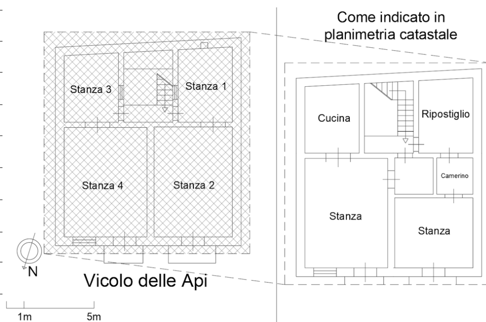
Figura 12: Planimetria della situazione reale dei luoghi relativa ai beni pignorati Lotto C, con evidenziate le difformità riscontrate rispetto alla situazione rappresentata nella planimetria catastale.
