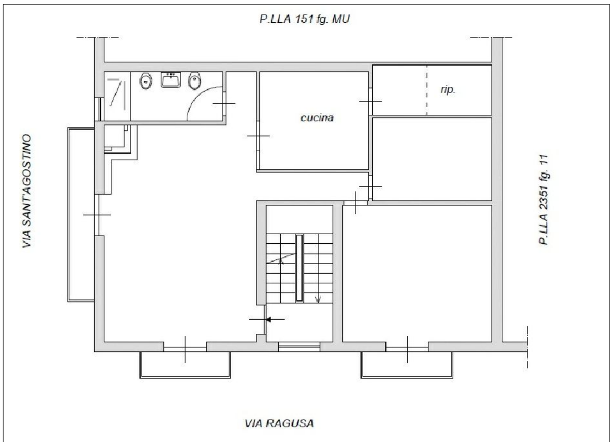
Planimetria dello stato dei luoghi
