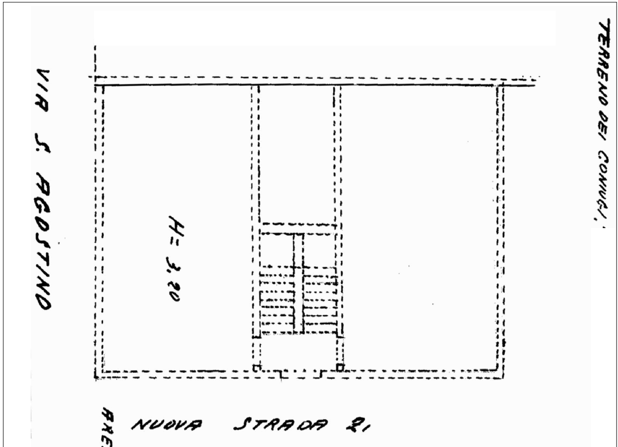
Planimetria catastale
