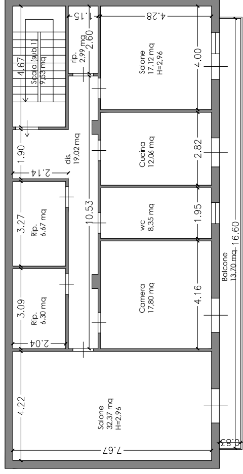
Planimetria piano primo
