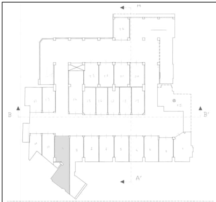
Fig. 30- Estratto del grafico di progetto della concessione del 2009 con indicazione del sub. 42
