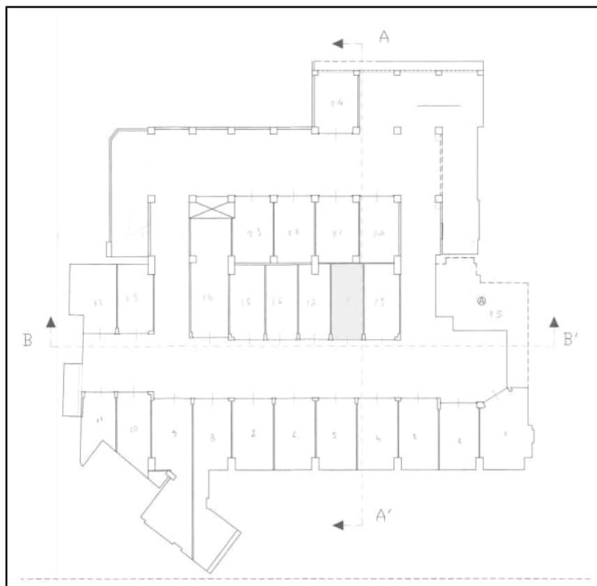
Fig. 30- Estratto del grafico di progetto della concessione del 2009 con indicazione del sub. 33
