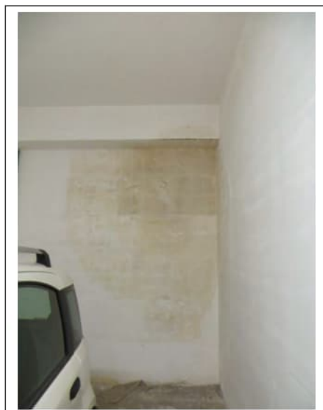
Fig. 27. Primo piano seminterrato. Box auto pignorato identificato al sub. 33. Degradi sulla parete di fondo
