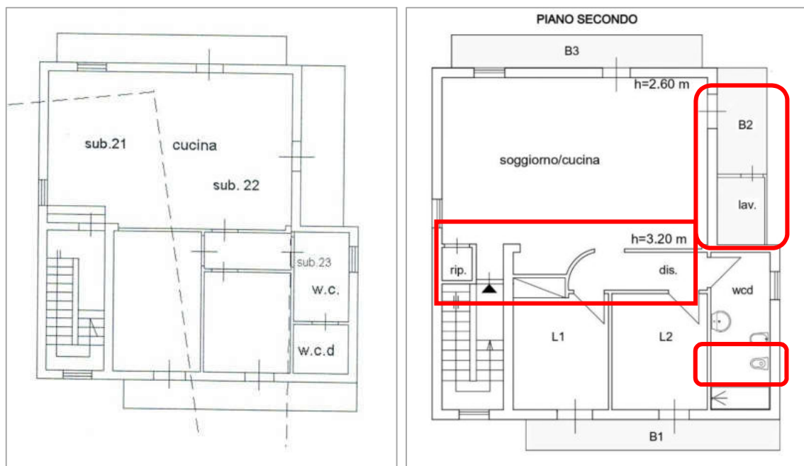
Fig.7 – Raffronto tra planimetria catastale e planimetria reale
