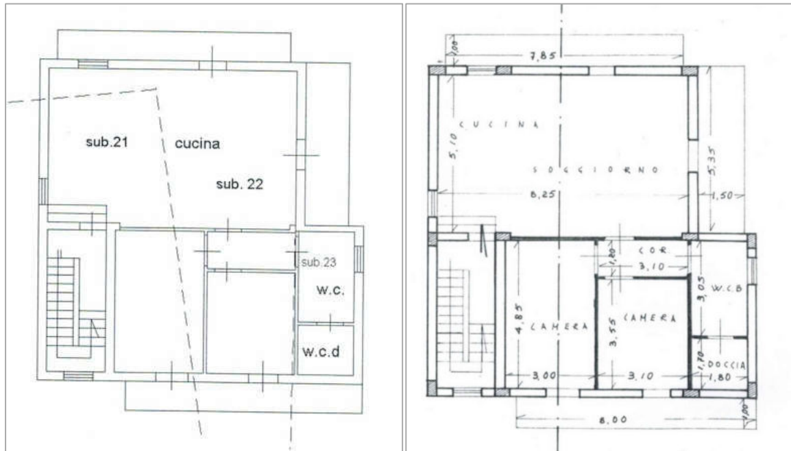
Fig.8 – Raffronto tra planimetria catastale e planimetria di progetto
