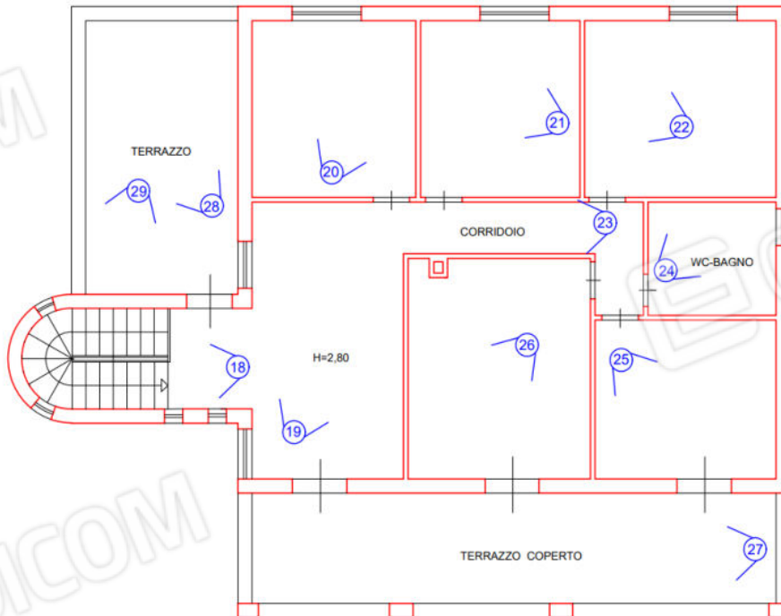
Planimetria dei coni ottici del villino-Piano primo.
