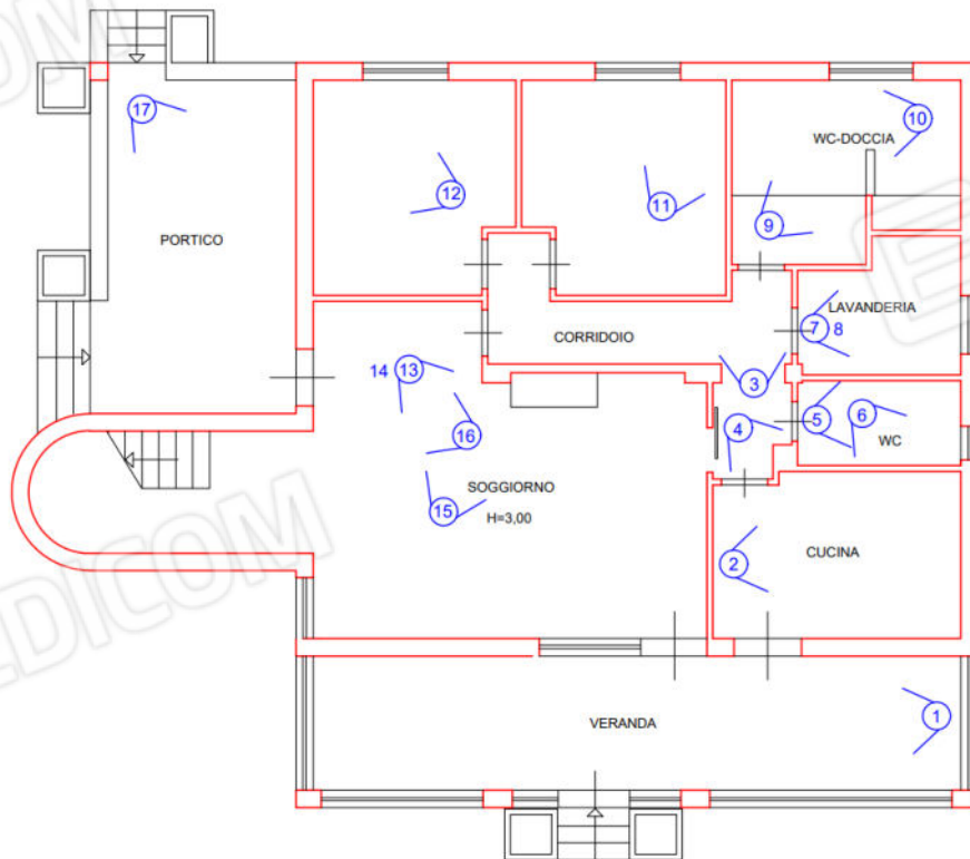
Planimetria dei coni ottici del villino-Piano terra
