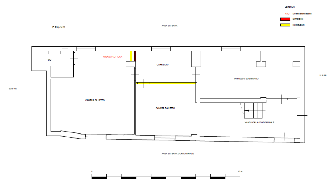
Planimetria di rilievo attuale con indicazione delle eventuali difformità rispetto alla planimetria catastale allegata al certificato di agibilità
