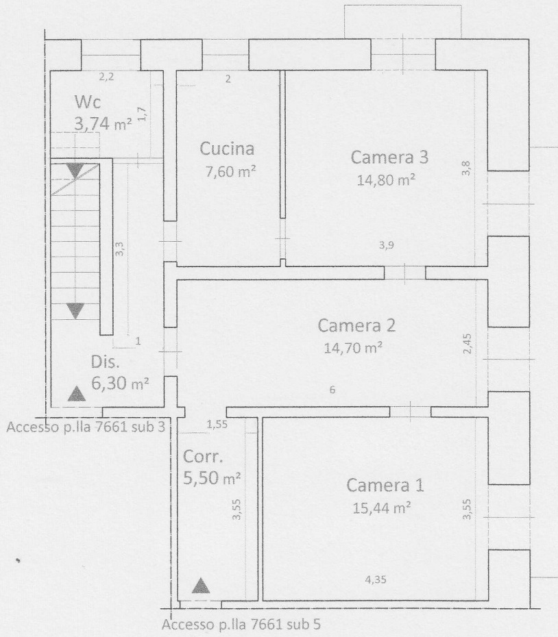
PIANTA 1°P
