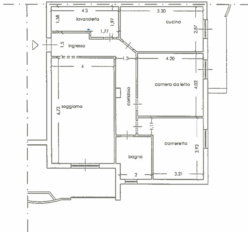
Piano Primo_Stato di Fatto_scala 1:100 rilievo effettuato in data 20/12/2023_Arch. Giuseppina CORSO
