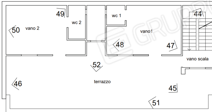
piano copertura
