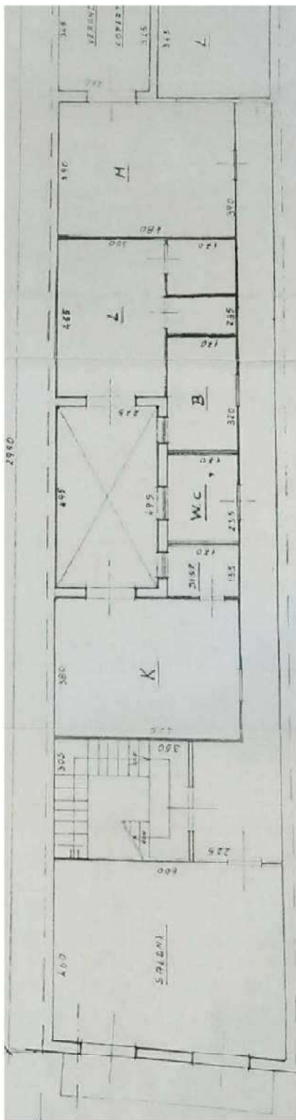
Planimetria primo e secondo piano - Concessione in Sanatoria n. 49 Rilasciata il 17/Maggio/1999
