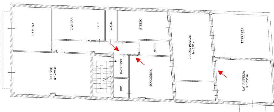
Pianta 1°P. (rilievo stato attuale) Prospetto Via Roma (stato attuale)
