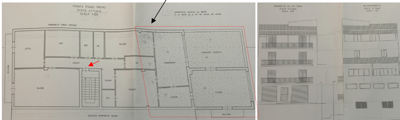
Pianta 1°P. (progetto U.T.C.)
