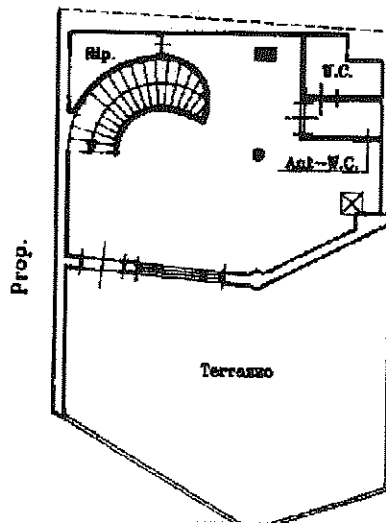
PIANO PRIMO RISTORANTE H= 3.10m.
