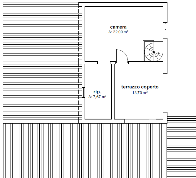
Pianta piano 1°
