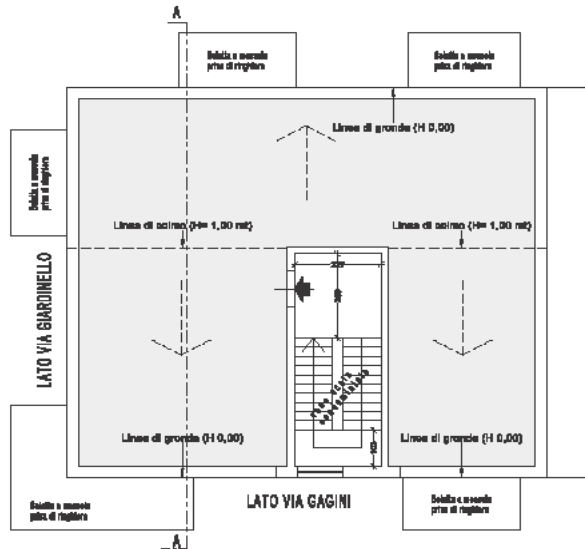
PIANTA SECONDO PIANO_LASTRICO SOLARE (sup. catast. mq 110)
