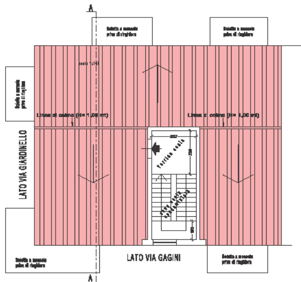
PIANTA DELLA COPERTURA DEL LASTRICO SOLARE (piano 2°)
