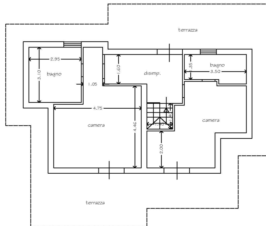
PIANO PRIMO/SOTTOTETTO
