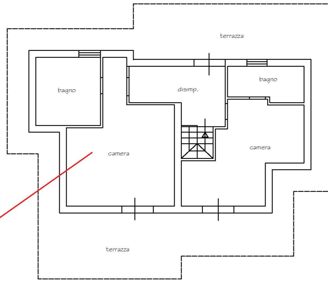
PIANO PRIMO/SOTTOTETTO
