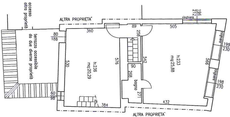
PIANO PRIMO
