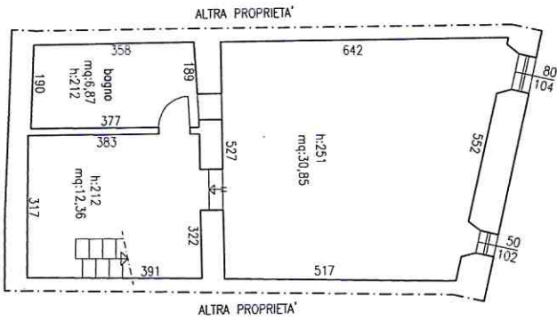
PIANO SOTTOSTRADA
