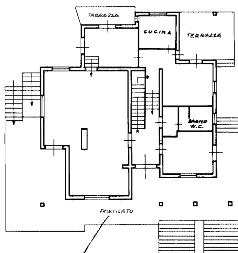
PIANO TERRA RIALZATO H: 3.00
