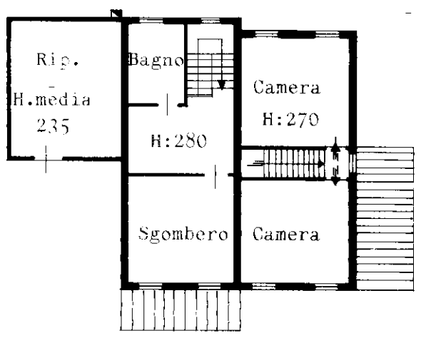
PIANO PRIMO
