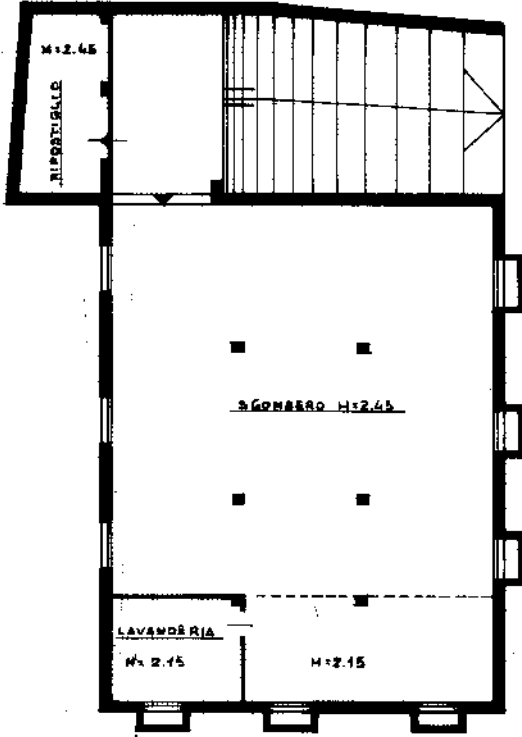
PRIMO PIANO SOTTOSTRADA
