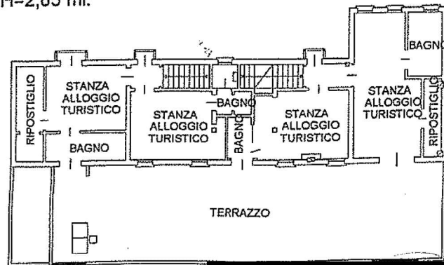
PIANTA PIANO PRIMO H=2,85 ml.
