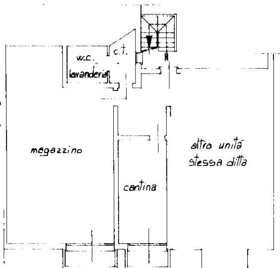
pianta piano interrato H=2.30
