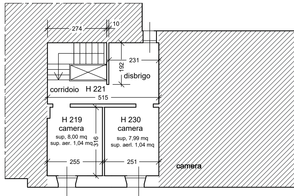
PIANO SECONDO
