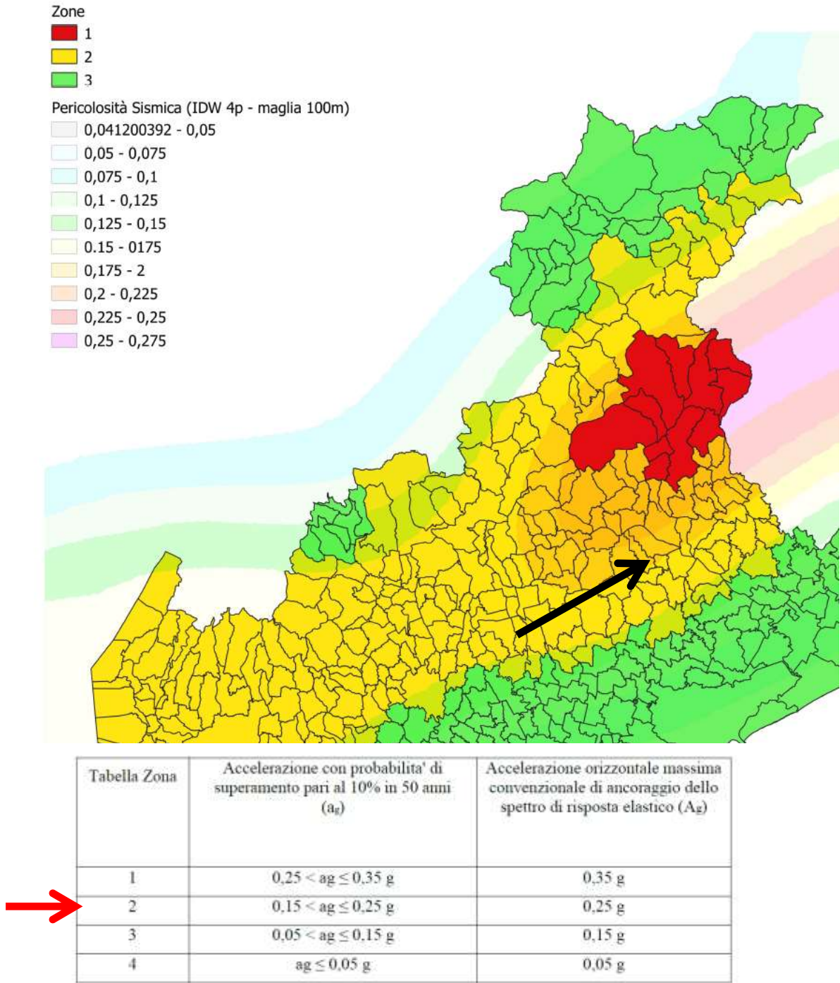
Fig. 7 – estratto della Zonizzazione Sismica di cui alla DRGV n. 244 del 09/03/2021 Classificazione sismica del Veneto Mappa di pericolosità sismica
