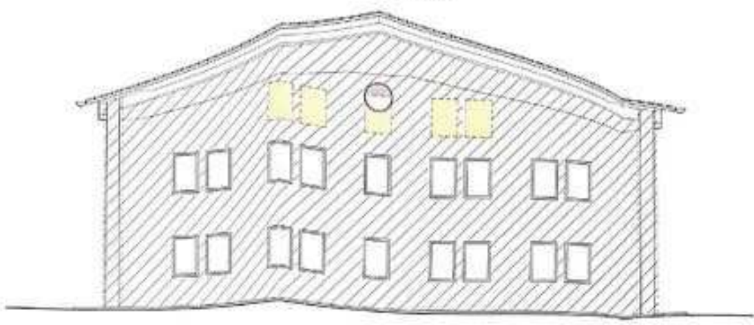
PROSPETTO NORD
