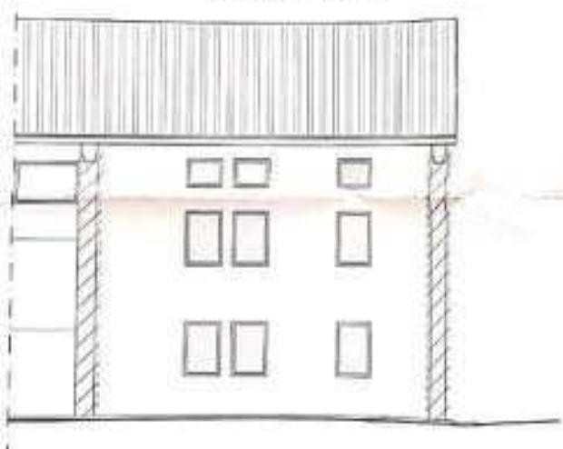
PROSPETTO EST
