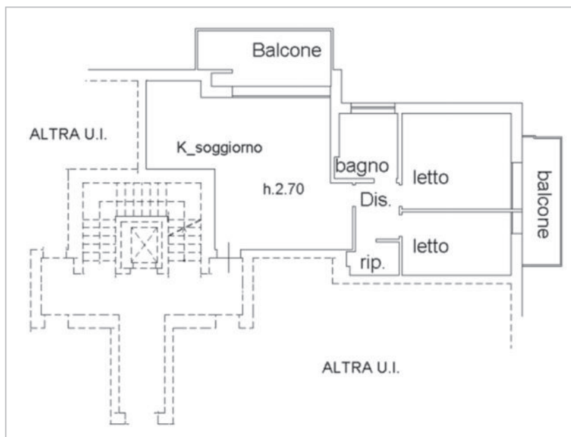
Planimetria appartamento sub. 7
