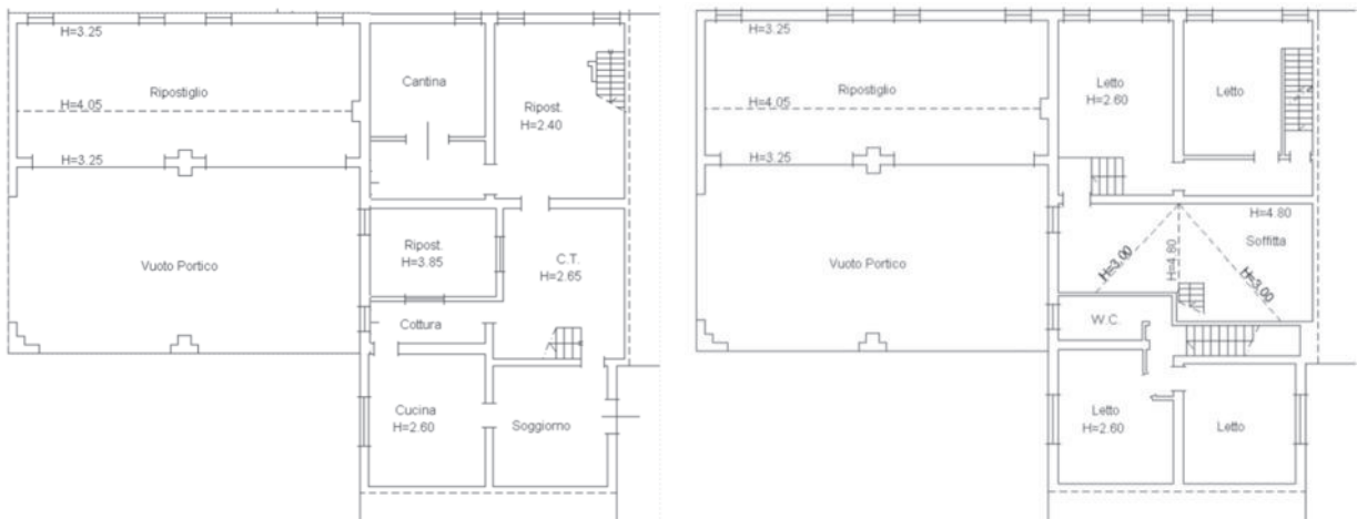
Planimetrie del piano terra e piano primo
