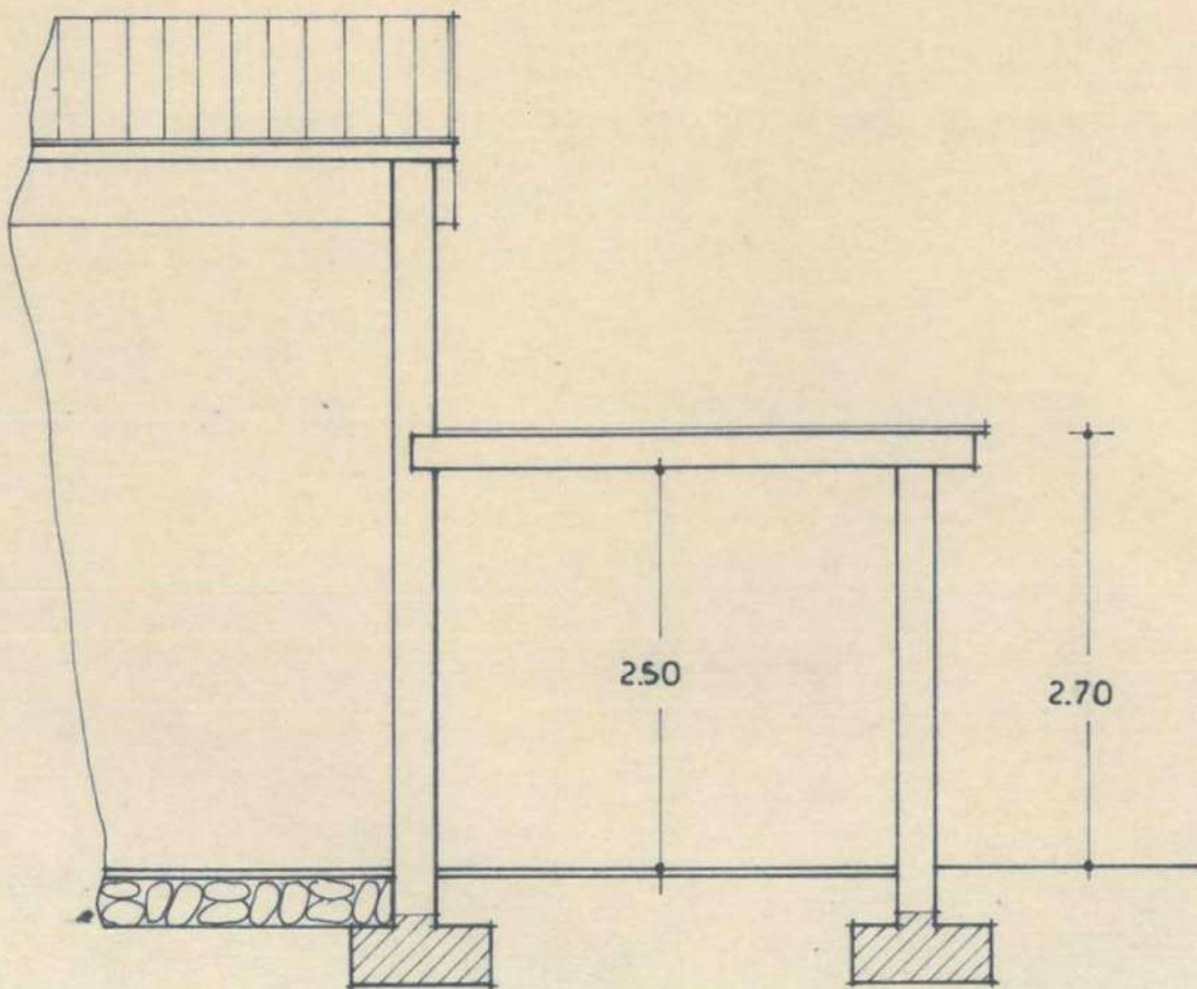
sezione aa
