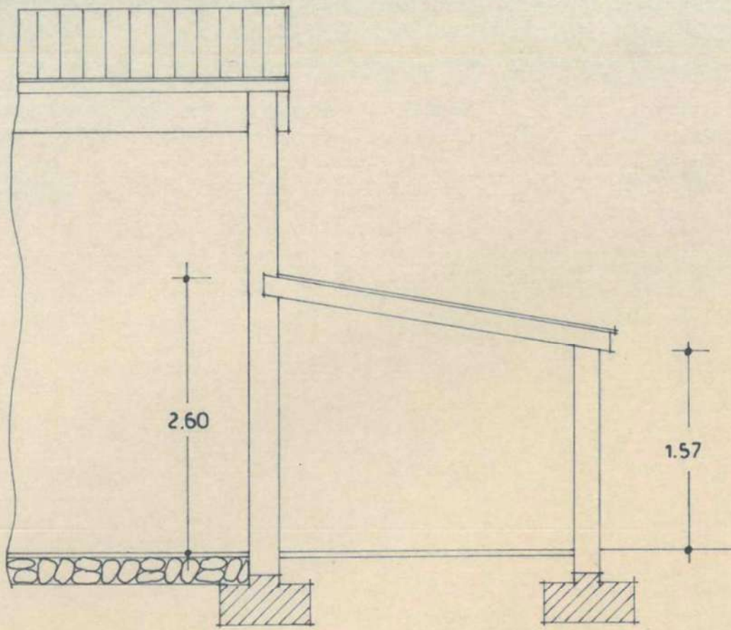
sezione aa
