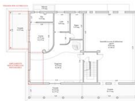
Stato di fatto - Piano primo
